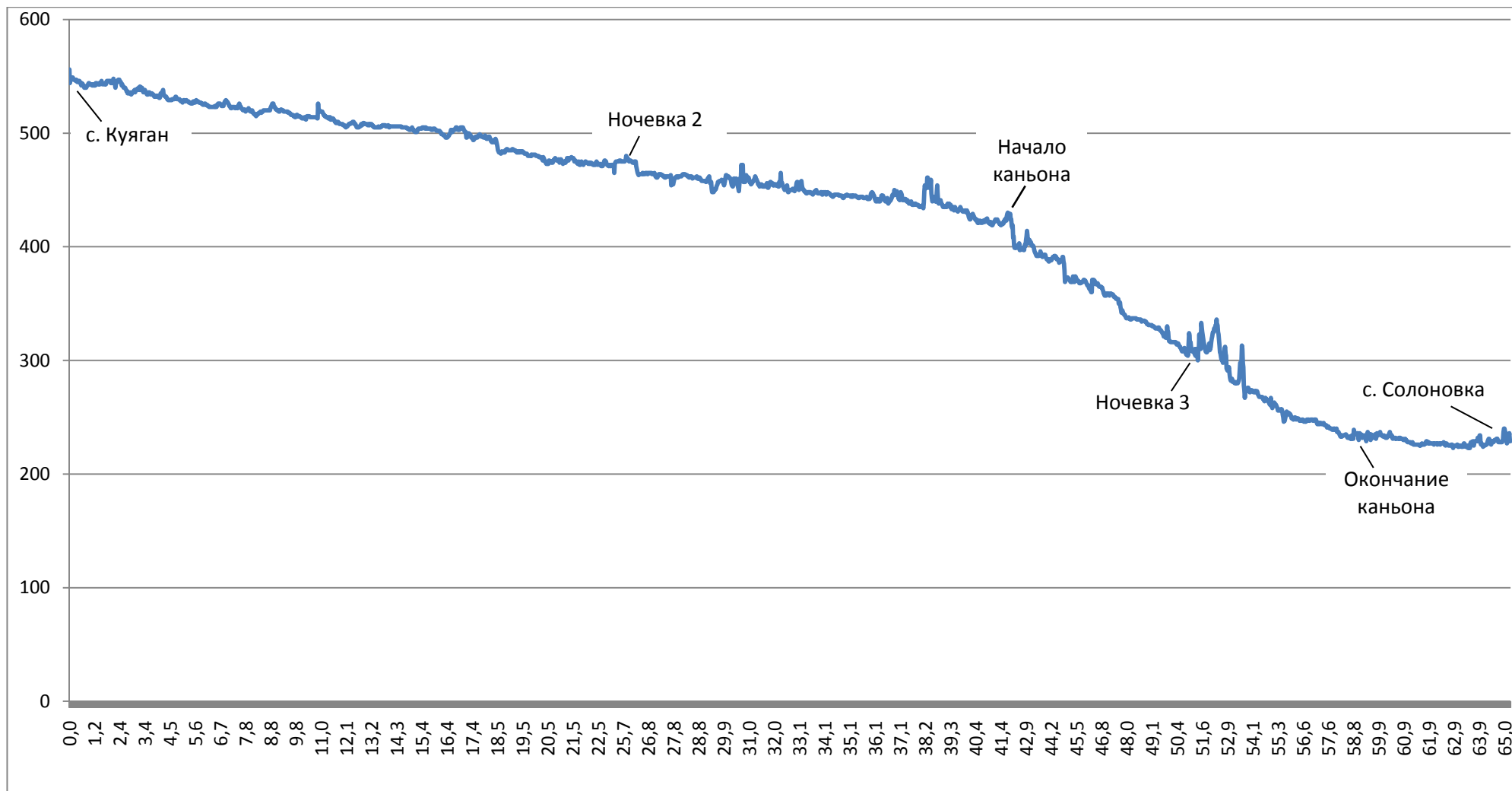
График зависимости уреза воды реки Песчаная в зависимости от расстоянийот с. Куяган до с. Солоновка
