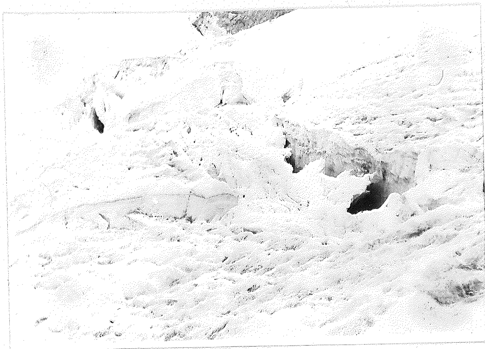
фото 23 . Трещины на леднике М.Ганза .
