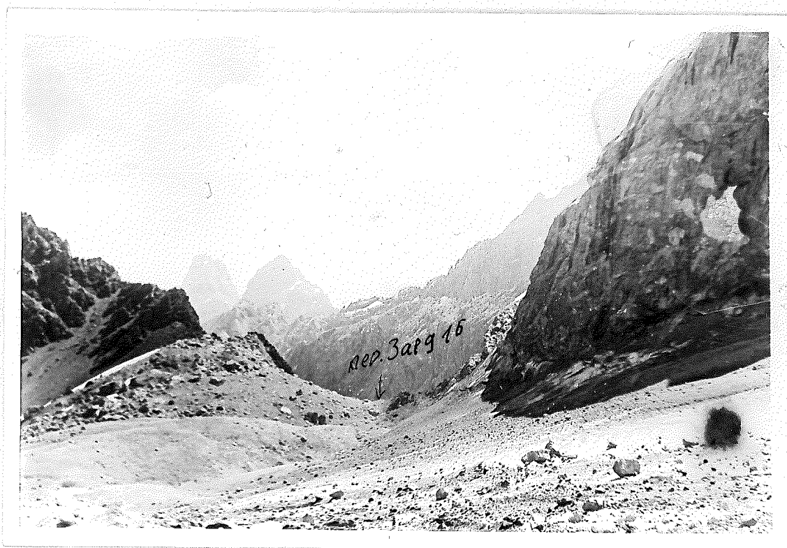
Фото 25 . Пер. Зард 16 со стороны р. Сурхоб .
