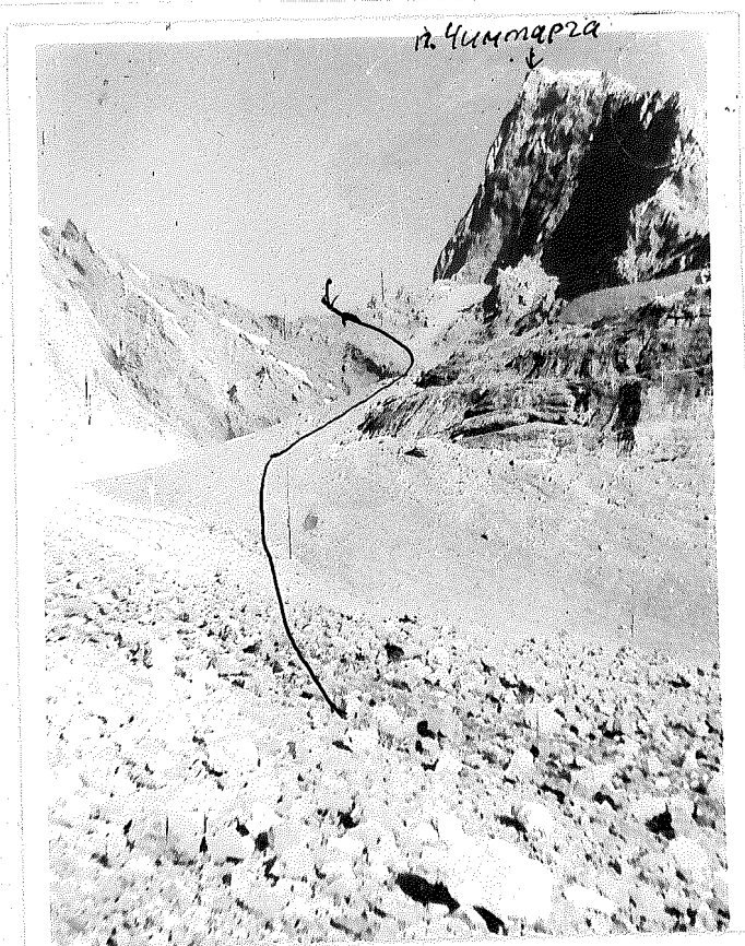
Фото 15 . Пер. Чимтарга 1Б со стороны Мутных озер . ( снято с пер. Казнок Зап. )
