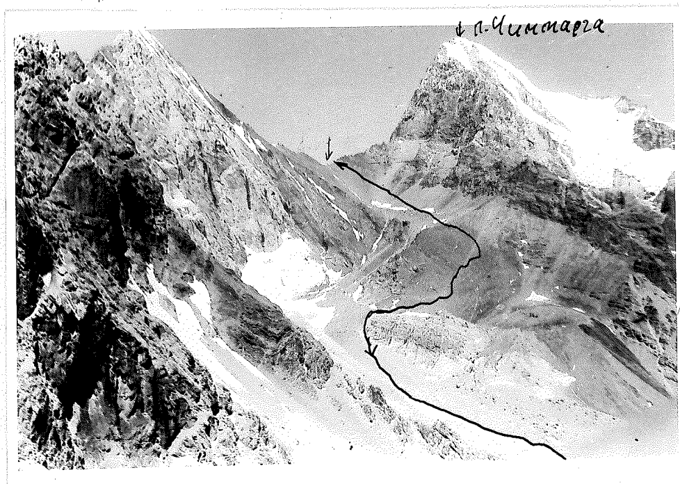
Фото 15 . Пер. Чимтарга 1Б со стороны Мутных озер . ( снято с пер. Казнок Зап. )
