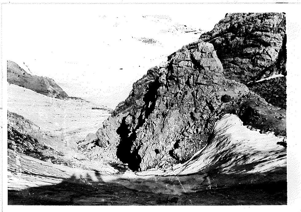
Фото 13 . Ледник на спуске с пер. Казнок Зап.2А .
