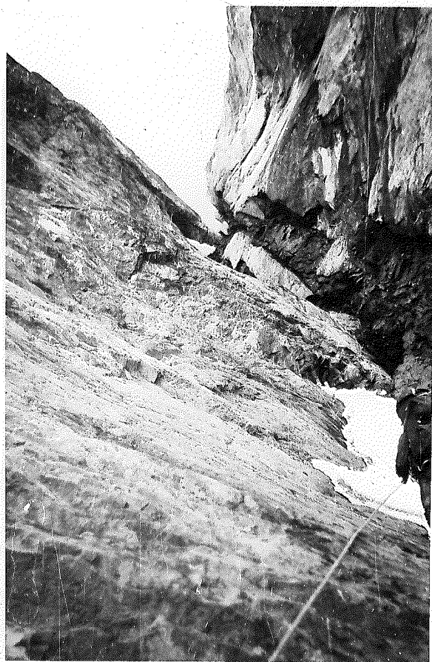
Фото 20 . Кулуар на пер. Юбилейный .
