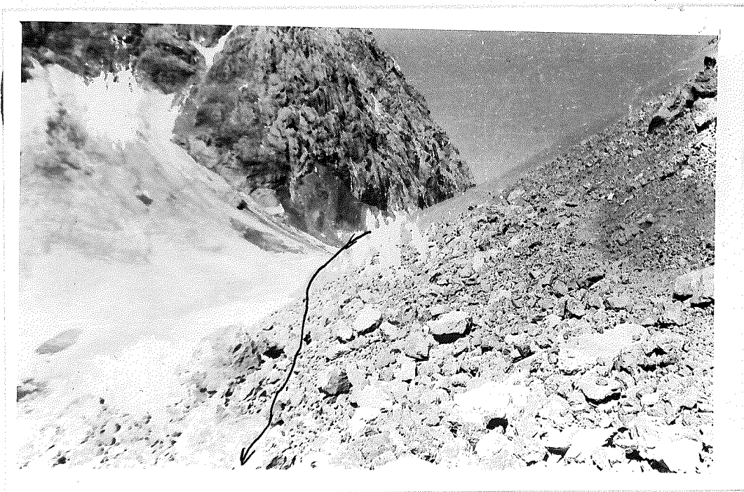
фото 6 . Пер. Дукдон 1А со стороны р. Дукдон .
