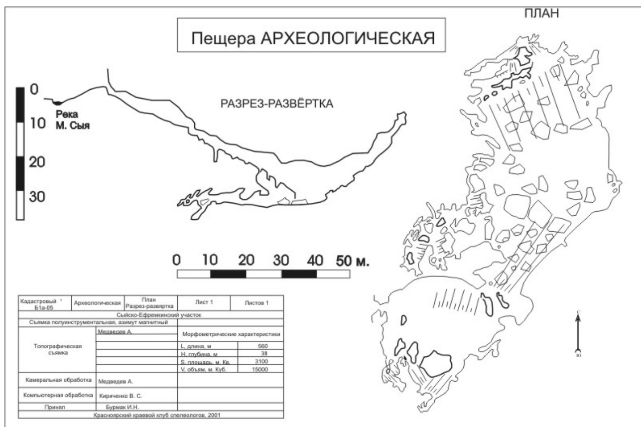
План и разрез пещеры Археологическая.
