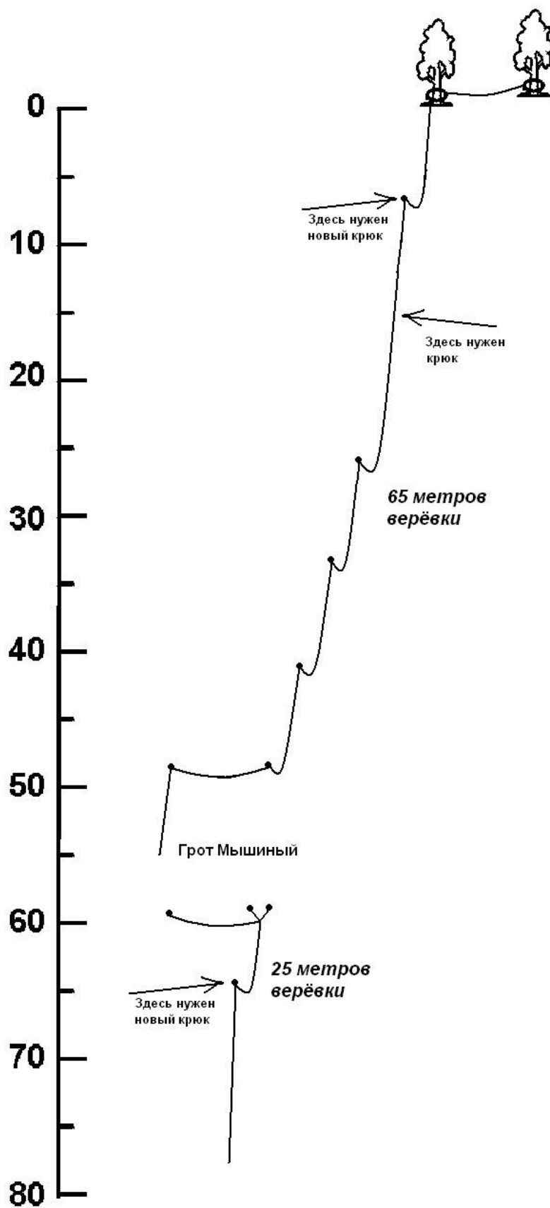
Схема SRT навески в пещере Виноградовская, по которой мы ходили.
