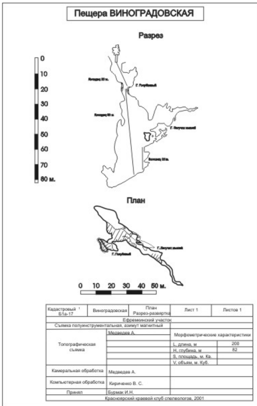
План и разрез пещеры Виноградовская.
