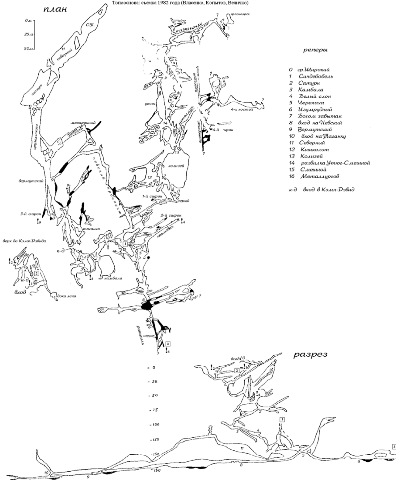
План и разрез пещеры Ящик Пандоры.
